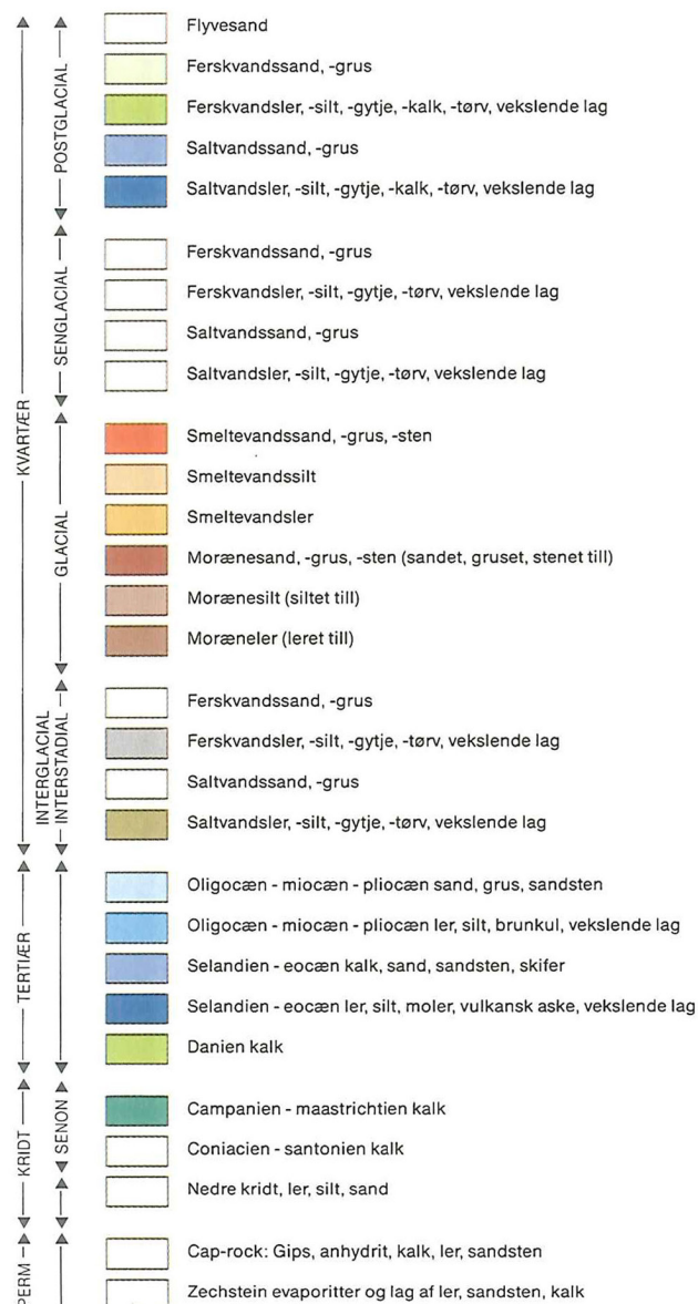
Figur 2. Farveinddeling for jordlag på basisdatakort
