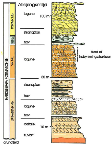
Figur 5. Lithostratigrafisk søjle over Hardeberga Formationen ved Vik.
