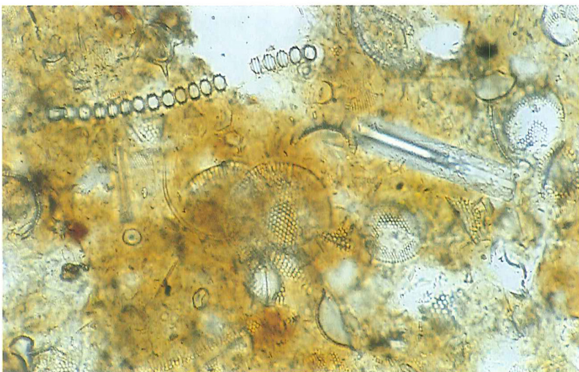
Figur 4. Vandret snit af den oligocæne diatomit. Forstørret.
