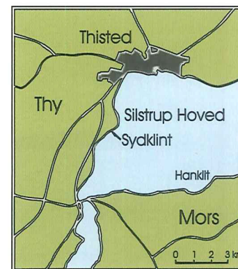
Figur 1. Klinerne ved Silstrup.
