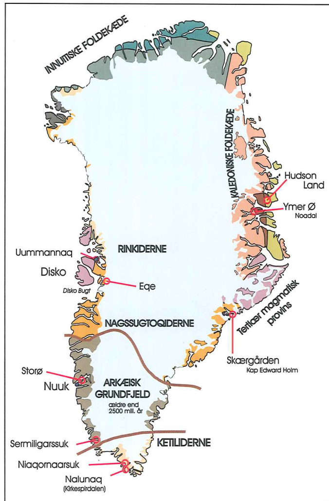
Geologisk oversigtskort over Grønland modificeret fra GGU kort. Artiklens guldkaliteter er angivet.
