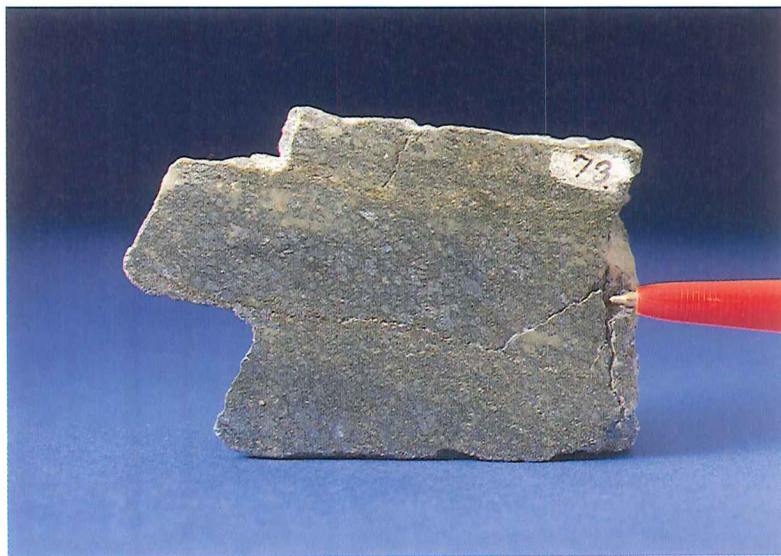
Guldførende bjergart med pyrit og arsenopyrit. Storø, Vestgrønland.
