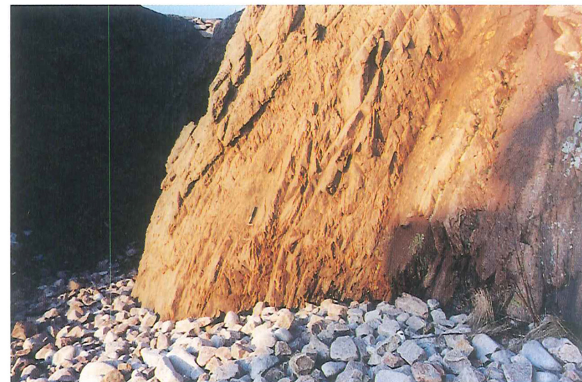
Figur 5. Kystklipperne i bunden af vigen visende tætliggende forkastningsplaner, der stryger ca. nord-syd og hælder 60-70 grader mod vest. Mellem planerne ses øst-hældende forkløftninger, der sammen med forkastningsplanerne giver snittet 'stige-struktur'. Det synes som om de gennemgående planer er forkastningsplaner, langs hvilke den vestlige (venstre) del er sunket i forhold til den østlige. Blokkene i strandvolden er i hovedsagen normal Hammergranit. Ikke en eneste blok af breccieret Hammergranit fandtes her.
