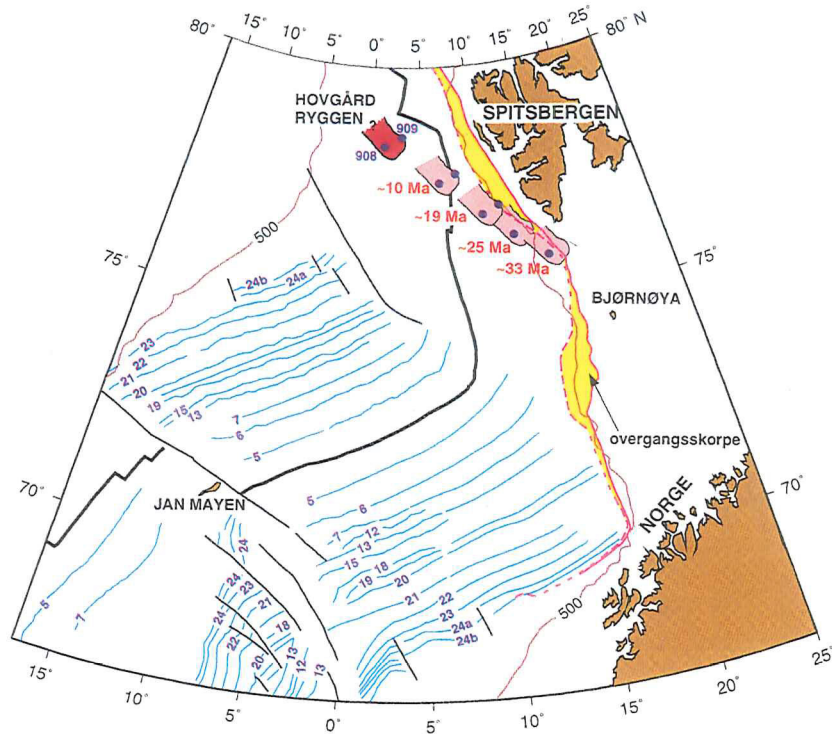
Figur 3. Hovgårdryggens bevegelse relativt til Svalbardplattformen fra tidligste oligocen (ca. 33 millioner år) til nåværende posisjon. Borehullene 908 og 909 er markert. Hull 909 er ikke plottet før ca. 19 millioner år som er alderen til de eldste sedimentene på lokaliteten. Figuren viser også spredningsanomalier (blå linjer) og hovedlinjer i spredningsakser og bruddsoner (sorte linjer).
