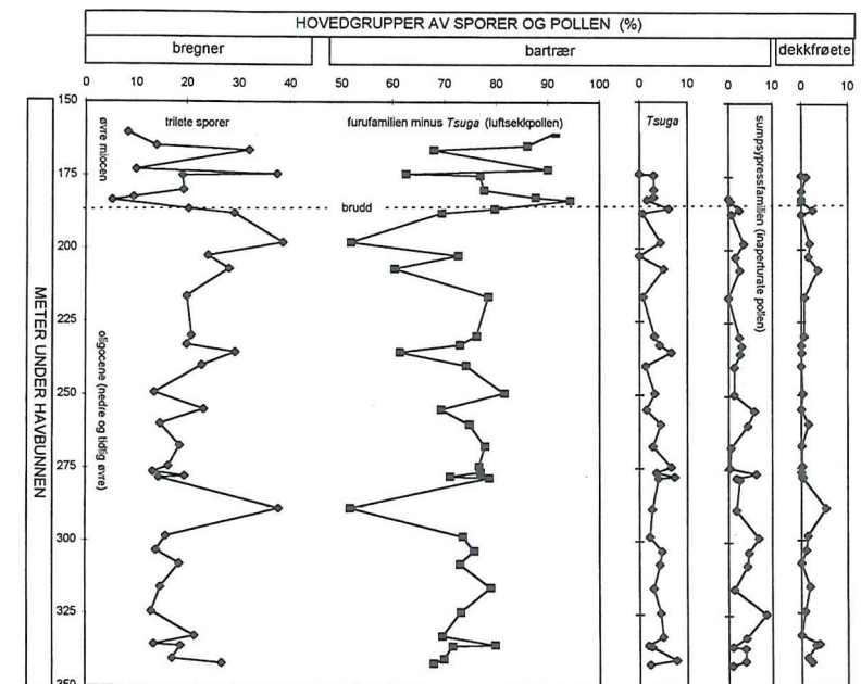
Figur 8. Pollendiagram hull 908. Diagrammet viser den relative andelen av bregnesporer (trilete sporer), luftsekkpollen av furufamilien, hemlockgran (Tsuga), inaperturate pollen (= pollen uden åbninger) (overveiende sumpsypress-familien), og dekkfrøete pollen.
