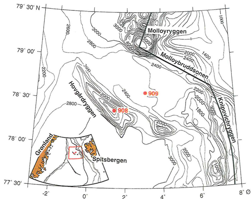
Figur 1. Den sentrale delen av Framstredet med Hovgårdryggen (havdyp i meter). Lokalitetene for borehullene 908 og 909 er markert samt de viktigste platetektoniske strukturene.
