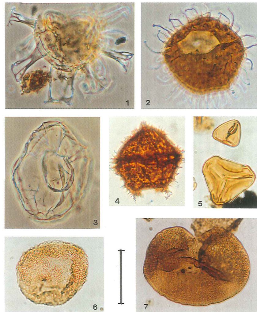
Figur 6. Eksempler på dinoflagellatcyster (1-4), sporer (5) og pollen fra Hovgårdryggens sediment (6: slekten hemlockgran, Tsuga ; 7: slekten gran, Picea ). Målestok = 5/100 mm (50 m).
