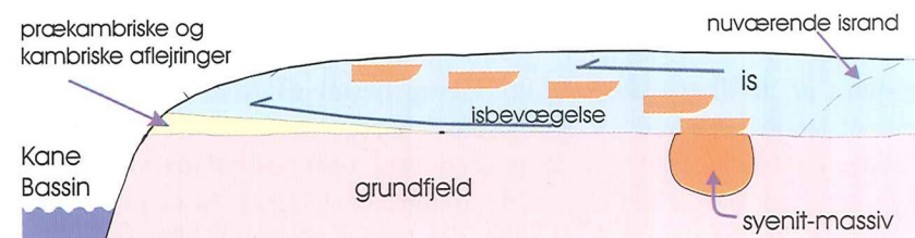
Figur 4. Profil (ikke i skala) gjennom Inglefield Land visende isens udbredelse under de første trin af dannelsen af Minturn cirklerne. Med punkteret streg er angivet den nuværende isrands placering. (Fra GEUS Årsberetning 1995).
