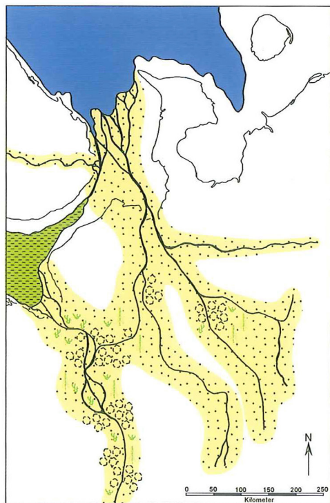
Tiden for 40.000-25.000 år siden. Isen er smeltet tilbage og på de store flodsletter dækker tundraen over permafrossen jordbund.
