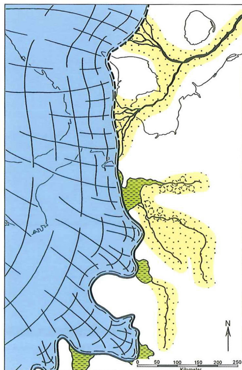
Tiden for 17.000 år siden. Den skandinaviske indlandsis når sin største udbredelse mod øst og opdæmmer samtidig en række mindre issøer foran gletscherfronten.
