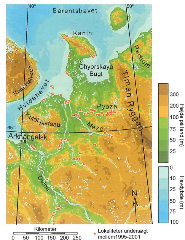
Arkhangelsk regionen, et område ca. 10 gange større end Danmark, med de lokaliteter vi har undersøgt siden 1995 og som danner grundlag for de efterfølgende kort. Kortgrundlag fra Jakobsson, 2000.
