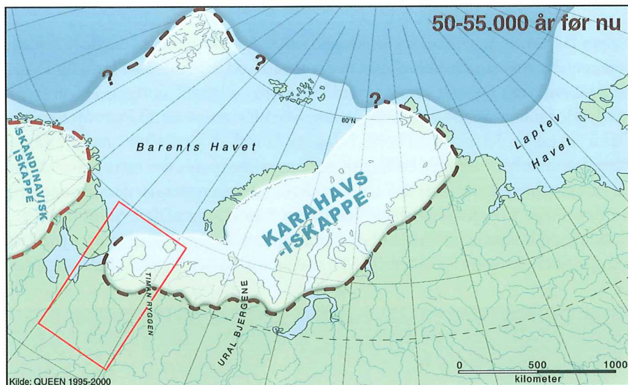
Karahavs iskappen for 55.000-50.000 år siden. Et mere detaljeret billede over Arkhangelsk regionen i denne periode er vist på forrige side.
