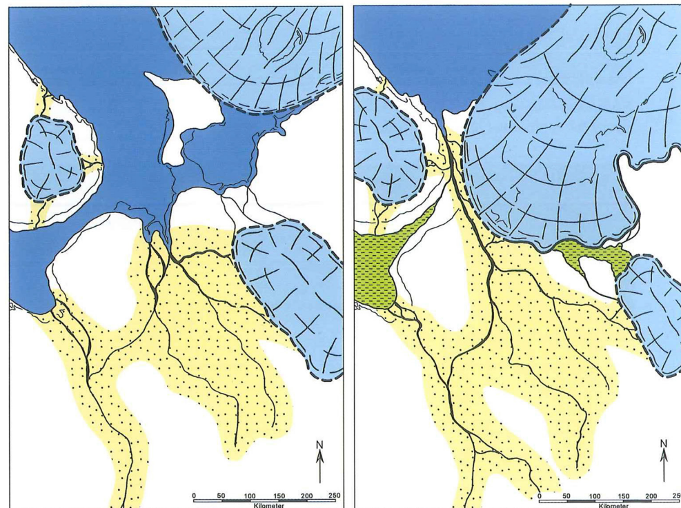
Tv.: Tiden for 60.000 år siden. Timan iskappen smelter, Karahavs iskappen glider frem og havet erobrer dele af Hvidehavskysten.
