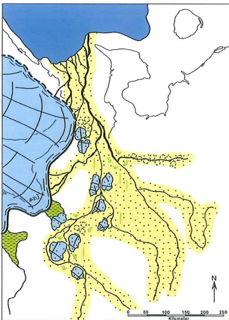
Tiden for 15.000-12.000 år siden. Den skandinaviske indlandsis er under tilbagesmeltning og efterlader dødis i lavliggende områder. Der er et kortvarigt ophold i denne tiltagesmeltning ved Hvidehavskysten.
