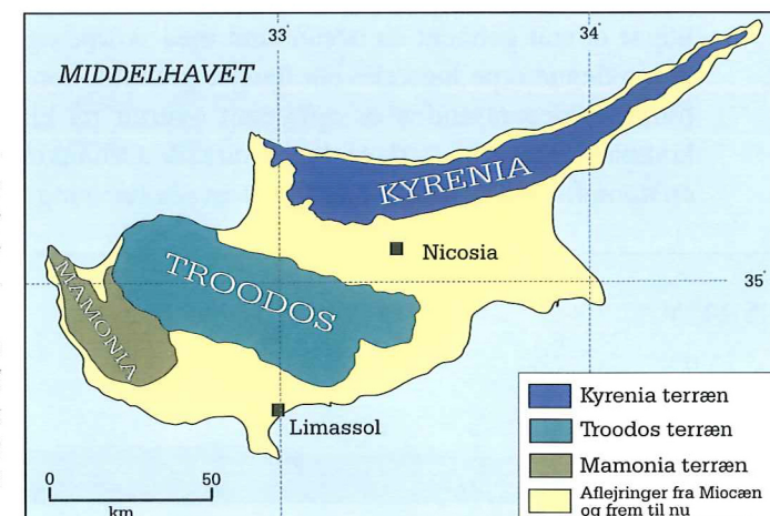
Figur 4. Geologisk skitse-kort af Cypern med de tre geologiske 'terræner', der danner baggrund for Troodos ofiolitkompleksets dannelse. Et geologisk 'terræn' er en distinkt tektonisk enhed med en bestemt geologisk historie – se teksten om sammensætningen af de viste terræner.
