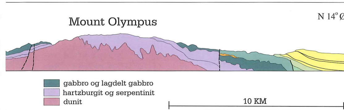
Figur 6. Profilsnit gennem det lagdelte og senere opdannede Troodos kompleks..
