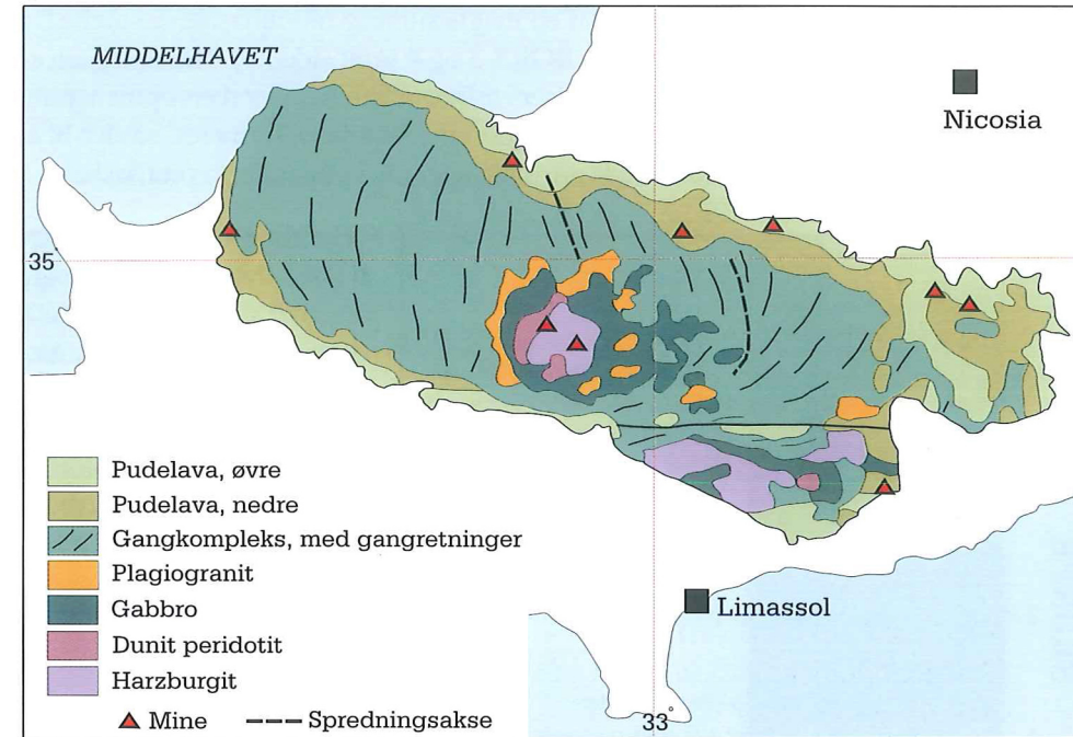
Figur 5. Geologisk oversigtskort over Troodos komplekset med angivelse af to fossile oceaniske spredningszoner, samt retning på gangintrusioner, der er parallelle med spredningsakserne. Blotningsmønstrets koncentriske form skyldes den sene domedannelse (se profilet gennem Troodos, figur 6), med en hævnning af den centrale del af komplekset.
