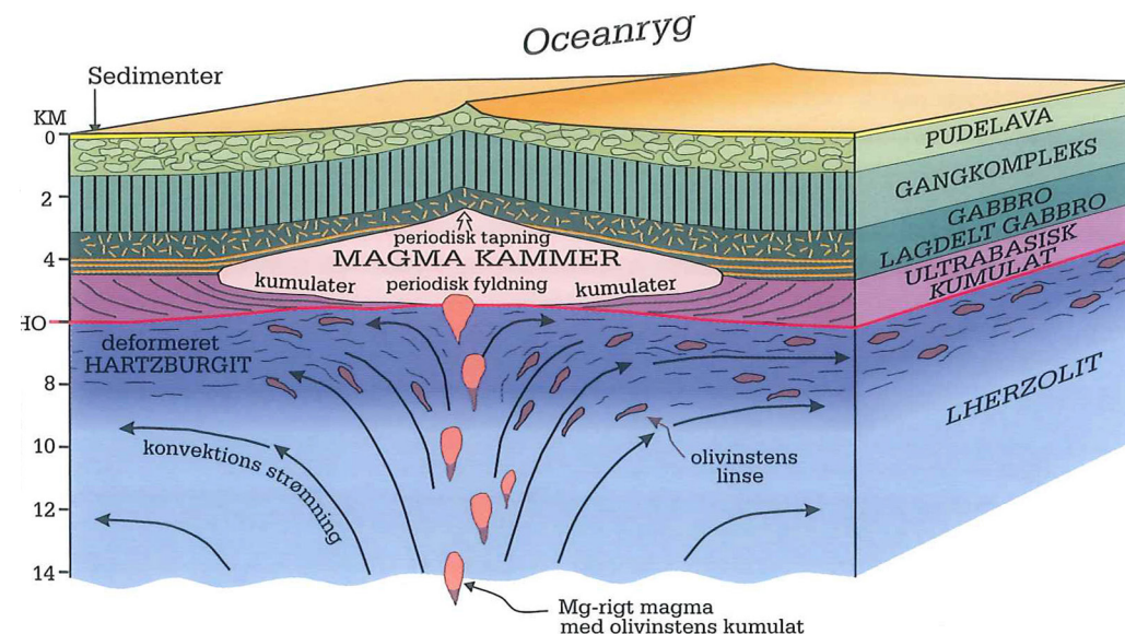
Figur 13. Blokdigram der viser en model for den tredimensionale opbygning af den øvre kappe og skorpen under en oceanisk spredningsryg, med en skematisk angivelse af de processer, der fører til dannelse af skorpebjergarterne.
