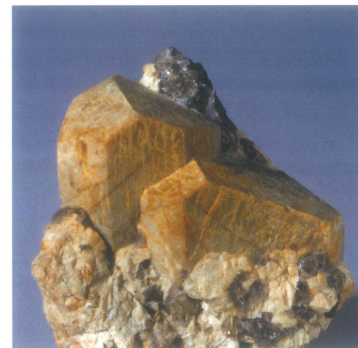
Figur 4. To kalifeldspat krystaller. Foto: O.B. Berthelsen
