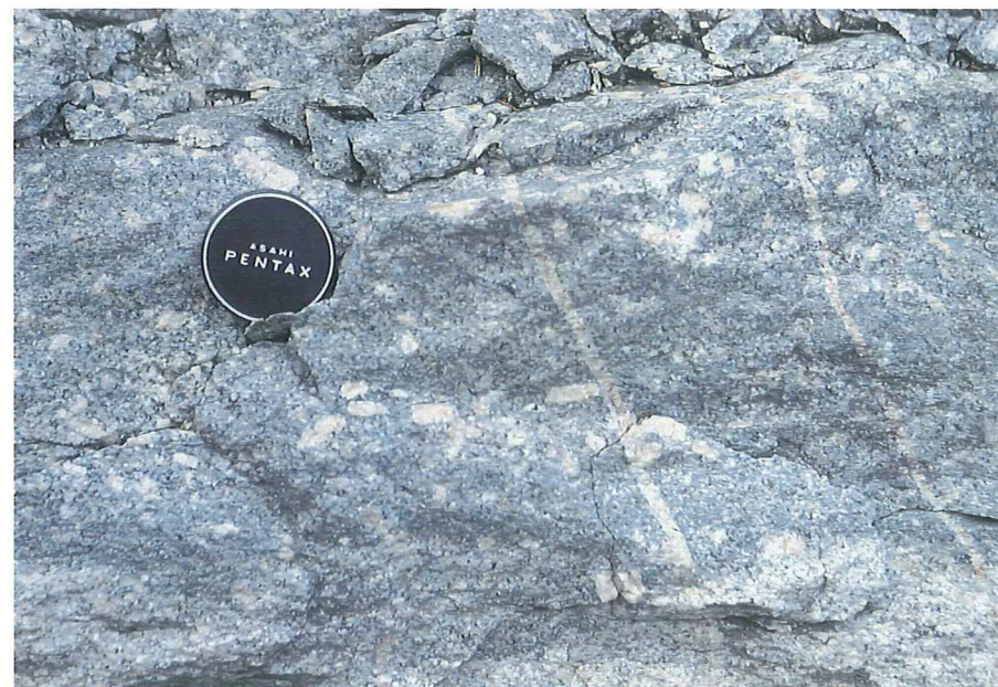
Figur 8. Hybridlignende bjergart dannet på grænsen mellem en grov granit og en gangformet monzonit.
