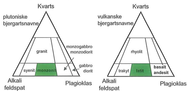
Streckeise's klassifikationsdiagram for magmatiske bjergarter med monzonit og granit indsat.
