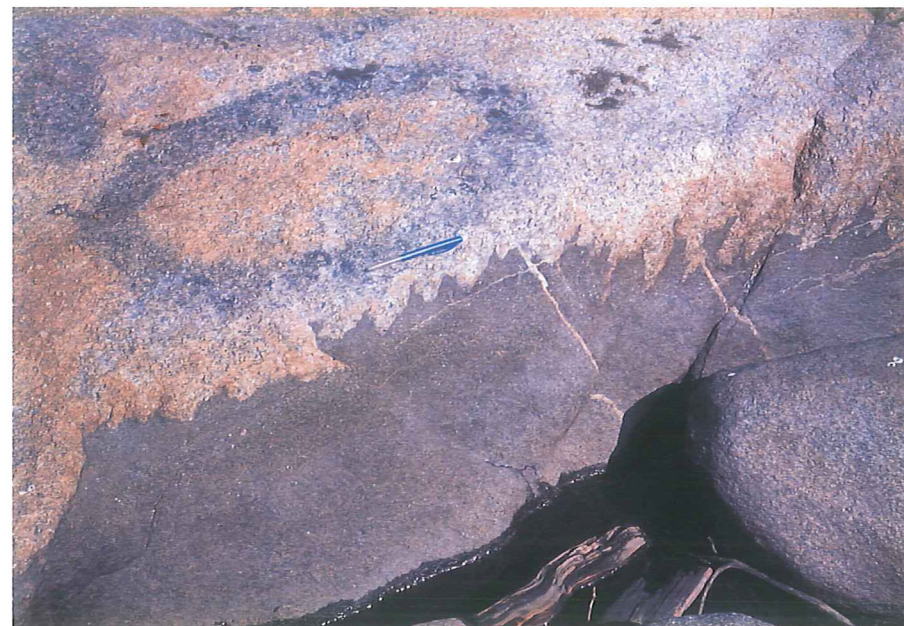
Figur 7. Uregelmæssig kontakt mellem monzonittisk gangbjergart og grovkornet granit.
