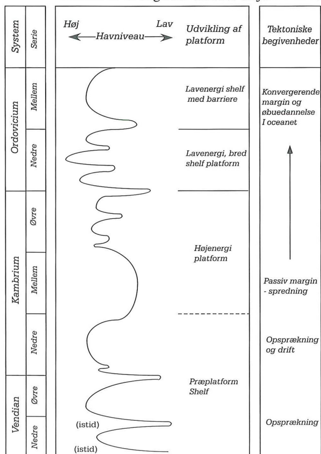
Figur 20. Sammendrag af udviklingen i Nordøstgrønland.
