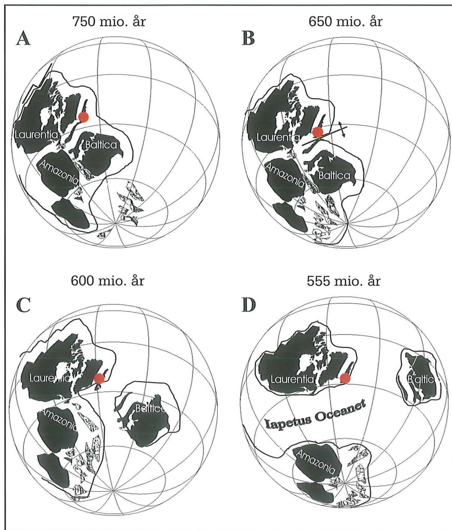
Figur 4. Prækambrisk palæogeografi:
