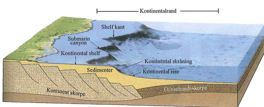
Figur 17. Den passive kontinentrand
