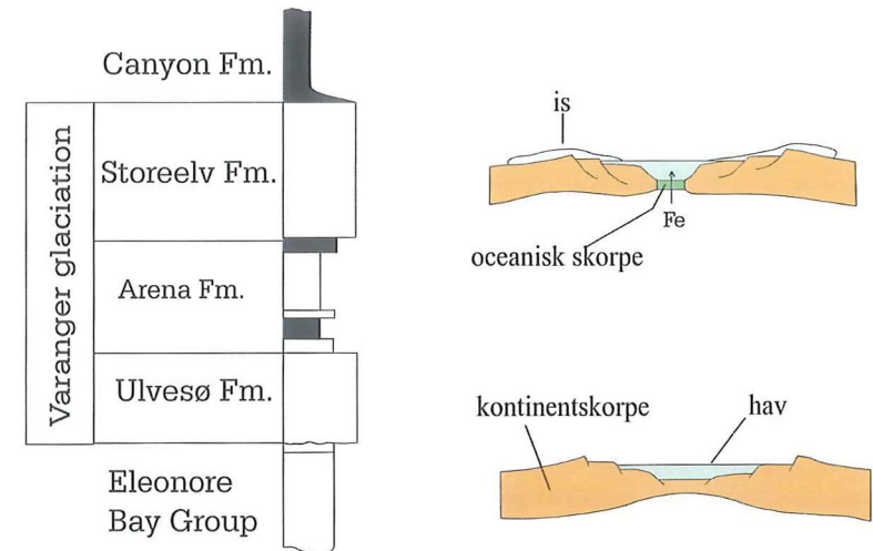
Figur 19. Jern(Fe)-berigelse af sedimenterne i øvre tillit (Storeelv Formation) på Ella Ø relateres til den første oceanbunds dannelse. Overgangen fra kontinental skorpe til tidlig drift og dannelse af oceanbund aflæses af Fe-indholdet. Dette er stigende i øvre tillit, idet Fe-rige hydrotermale opløsninger har beriget sedimenterne.
