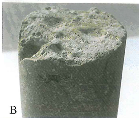
Figur 11. (a) En cylindrisk prøve af Midale Marly dolomit som den ser ud før et eksperiment. (b) Efter en måneds \text{CO}_2 -injektion ses der især i indløbsenden af prøven tydelig opløsning af bjergarten. Bemærk de små huller fra opløste mineralalkorn. Der observeres også en stigning i prøvens porøsitet og permeabilitet under strømnings-eksperimentet. Prøvens diameter er 2,5 centimeter. (C) Scanning elektron mikroskop billedet viser en typisk Marly dolomit med veludviklede dolomitmikrystaller (do) samt lidt accessorisk alkalifeldspat (af) og pyrit. (D) Efter \text{CO}_2 -injektion er dolomit-krystallerne markant ætsede i indløbsenden, med en karakteristisk udvikling af udhulede krystaller. (C) og (D) er i samme skala (GEUS Kerne Laboratorium, 2003).
