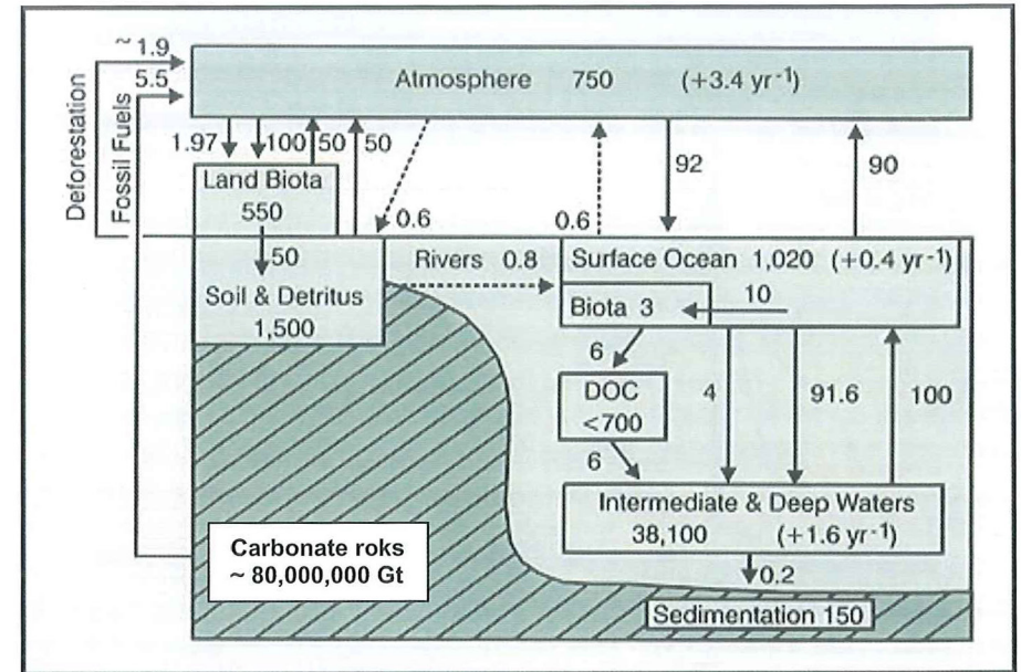
Figur 3. Det nutidige kulstofkredsløb for systemet atmosfære-ocean-kontinent i gigatons kulstof/år ( GtC/year ). Bemærk at kulstoflige vægten atmosfære-ocean er forskudt ca. 50 gange mod oceanet. Denne tendens gælder også for CO_2 . Havet fungerer derfor som en stor stødpude for CO_2 , men er alligevel ikke i stand til at optage hele den overskydende mængde CO_2 , som årligt tilføres atmosfæren. DOC=dissolved organic carbon (IPCC, 1996).
