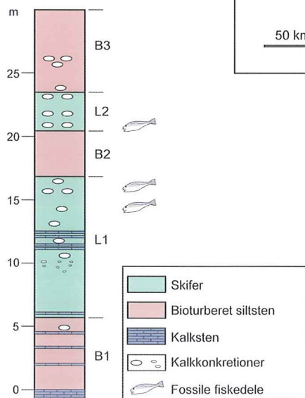
Figur 10. En sedimentologisk log der viser den typiske litologiske fem-deleling af Ravnefjeld Formationen. Der blev ofte fundet fossiler af fisk inden i de mange kalkkonkretioner.
