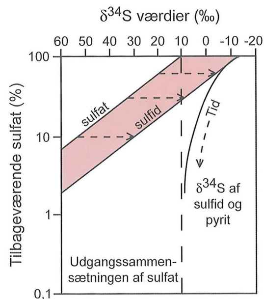
Figur 5. Dette Rayleigh-diagram viser, hvorledes den isotopiske sammensætning ændres i de udfældende og residuale faser med tiden. Hvis der er tale om et lukket system uden tilførsel af sulfat vil isotopsammensætningen af den sidst udfældende mineralfase være beriget på ^{34}\text{S} i forhold til udgangssammensætningen af havvandssulfat-svovl.
