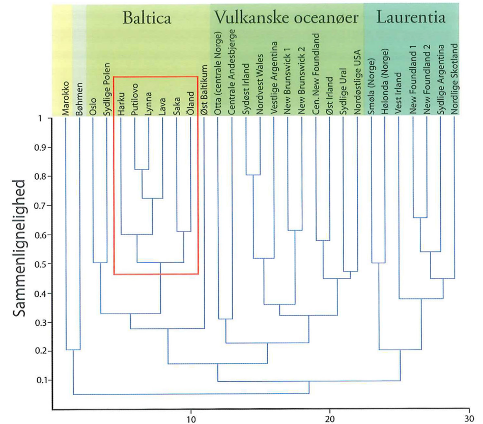
Figur 12. Cluster analyse visende sammenligneligheden mellem brakiopodfaunaer fra lokaliteter på forskellige palæokontinenter i Mellem Ordoviciem. Materialet, der ligger til grund for denne undersøgelse, er markeret i den røde firkant. Som det ses af diagrammet, grupperer de undersøgte lokaliteter sig tæt op ad de andre baltiske lokaliteter.
