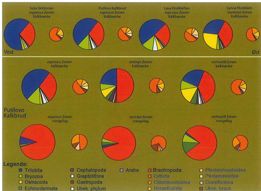
Figur 8. Fordelingen af den relative faunasammensætning i de undersøgte biozoner. De fire øverste – store - diagrammer viser variationen langs det undersøgte profil, mens de nederste seks – store - diagrammer viser variationen i de to forskellige litologier; hhv. kalk og mergel, i Putilovo kalkbrud. Det indbyrdes forhold af brakiopodgrupperne, hvis navne er angivet med blå skrift i signaturforklaringen, er vist i de små cirkeldiagrammer. Se Boks 2 for en kort gennemgang af dyregrupperne.
