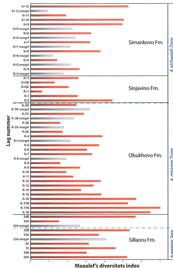
Figur 14. Den lagvise fordeling af Magalef's diversitets index i Putilovo Kalkbrud målt på brakiopoder. Rød farve angiver kalklag, mens grå farve indikerer mergellag. Lito- og biostratigrafiske enheder er angivet i højre side af diagrammet.
