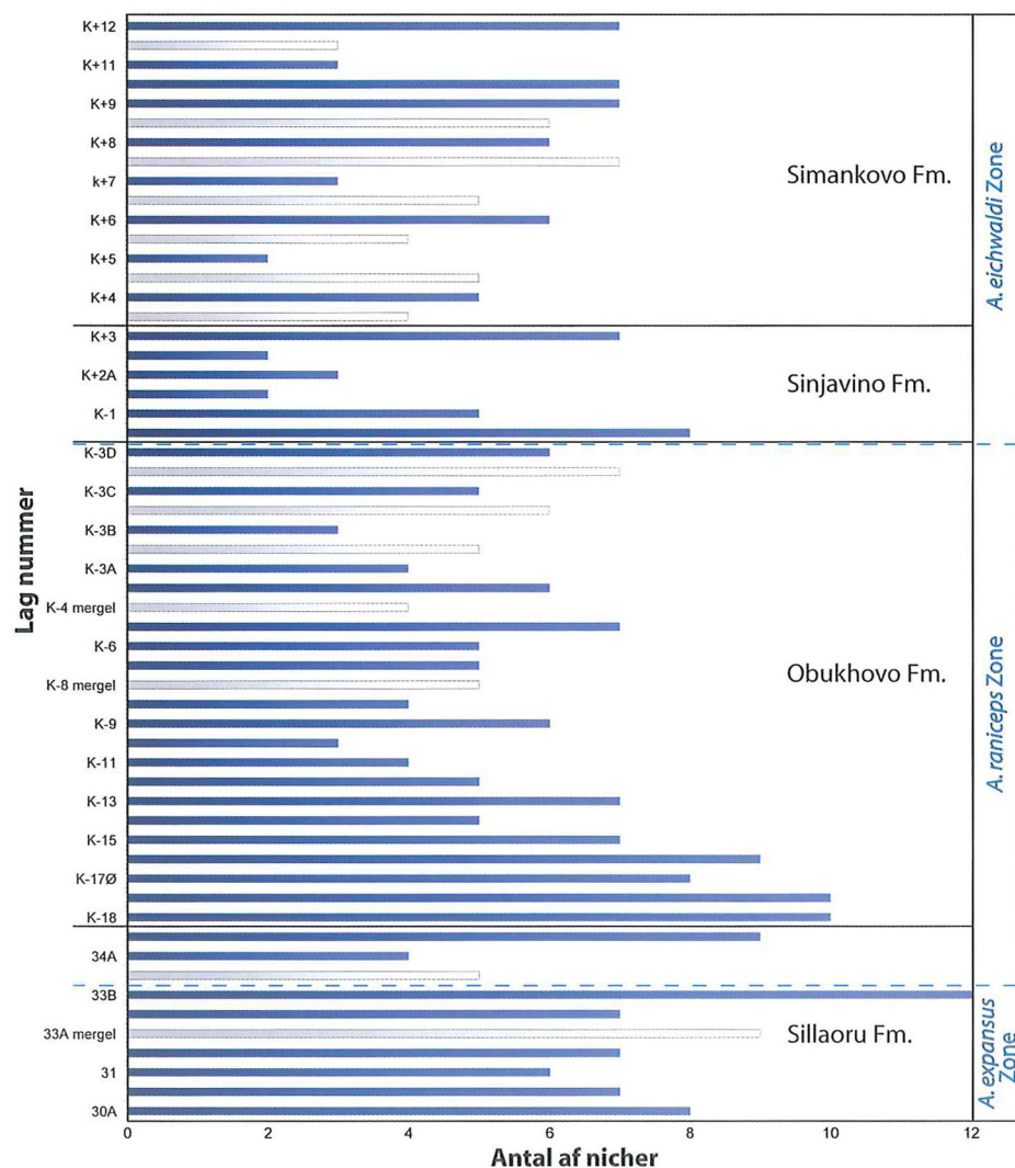
Figur 16. Brakiopodernes lagvise udnyttelse af de økologiske niches i Putilovo Kalkbrud. Blå farve angiver kalklag, mens gråhvid indikerer mergellag. Lito- og biostratigrafiske enheder er angivet i højre side af diagrammet.
