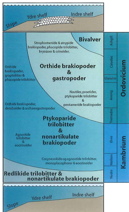
Figur 10. Den bassinverds forskydning af dyregrupper, der er karakteristiske for de tre evolutionære faunaer gennem Kambrium og Ordovicium samt gruppernes placering i forhold til et siliciklastisk (nederst) og et karbonat (øverst) shelfprofil. For trilobitter og brakiopoder er desuden angivet udviklingen for nogle væsentlige undergrupper. Endvidere kan nævnes, at dendroiderne er en orden inden for graptolitterne, archaeogastropoderne hører til gastropoderne og eocrinoiderne er en klasse af echinodermer.
