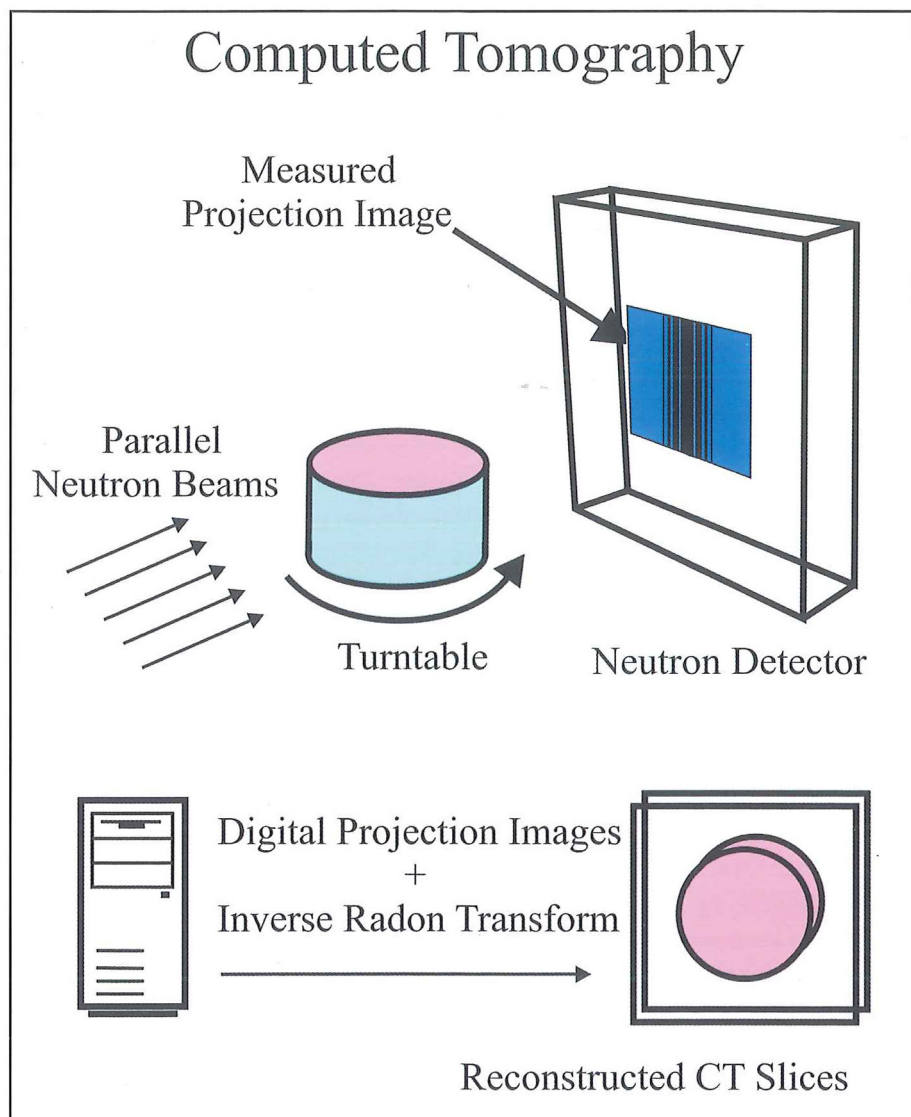
Figur 4. Princippet bag neutrontomografi taget fra Paul Scherrer Instituttet (PSI's) hjemmeside. Neutronstrålen kommer ind fra venstre, gennemlyser prøven, og der optages et billedet på en to-dimensional detektor. Prøven drejes en smule og processen gentages som regel flere hundrede eller tusinde gange. Den tre-dimensionale struktur kan derefter rekonstrueres med hjælp af rekonstruktionsalgoritmer og rå computerkraft.
